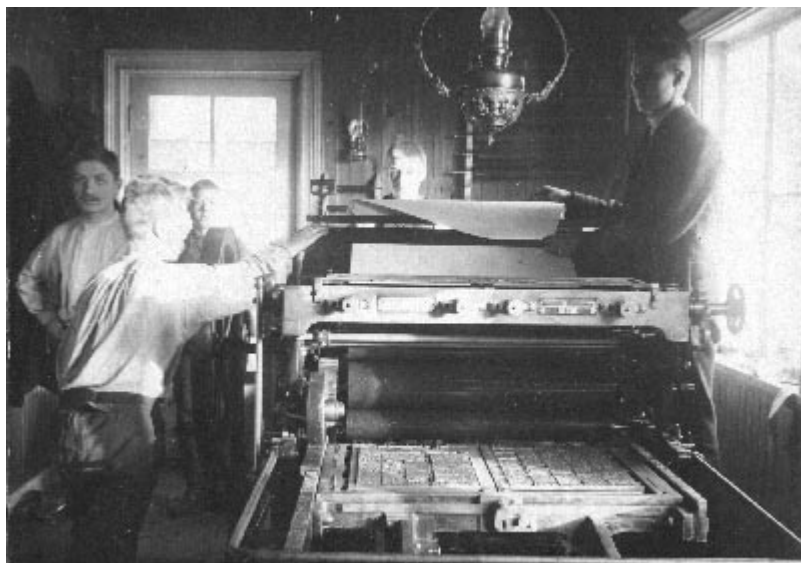
Työläinen-lehden kirjapaino Porvoossa 1913. Painokonetta väännetään käsin öljylamppujen valossa.
