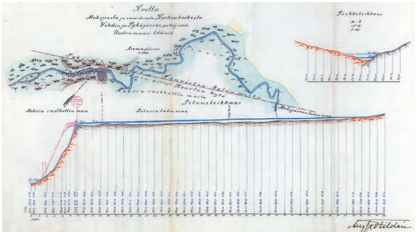
Aug. Fr. Hildénin laatima asema- ja pituusleikkauspiirros Korkeakosken padosta.
