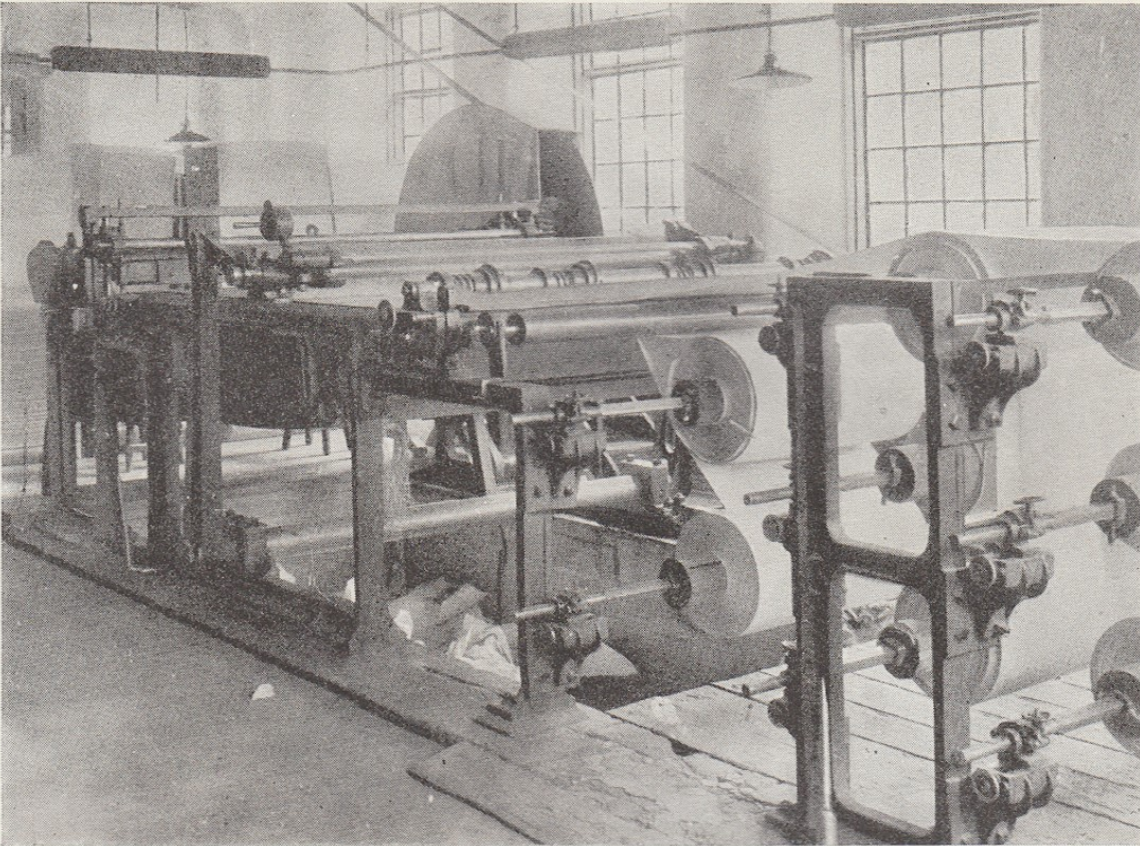
Paperin leikkuukone
