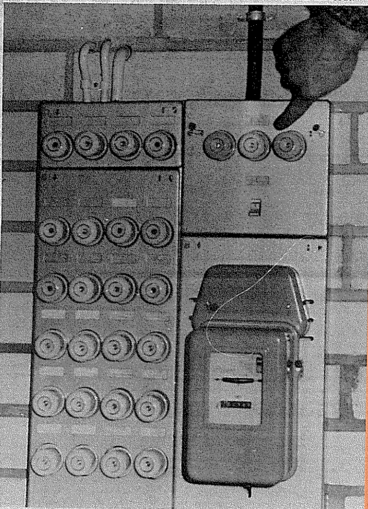
Sormi näyttää tavallisen sähkömittarin pääsulakkeen paikan.
