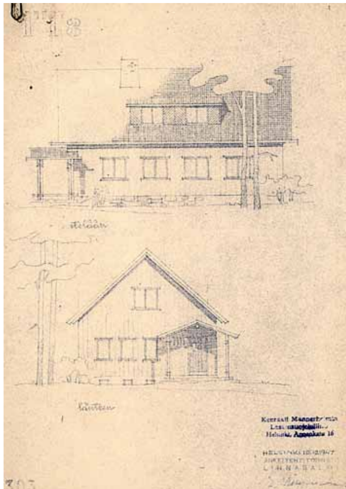
Nämä Erkki Linnasalmen TT3 tyyppiirustusten julkisivupiirustukset löytyivät MLL:n arkistosta. Näitä ei kuitenkaan merimaskussa noudatettu.
