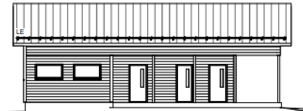
Julkisivu Länteen
