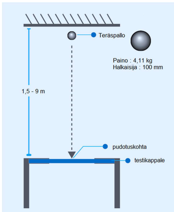
Kuva 8. Murtautumiskestävyden testaus teräskuulalla.
