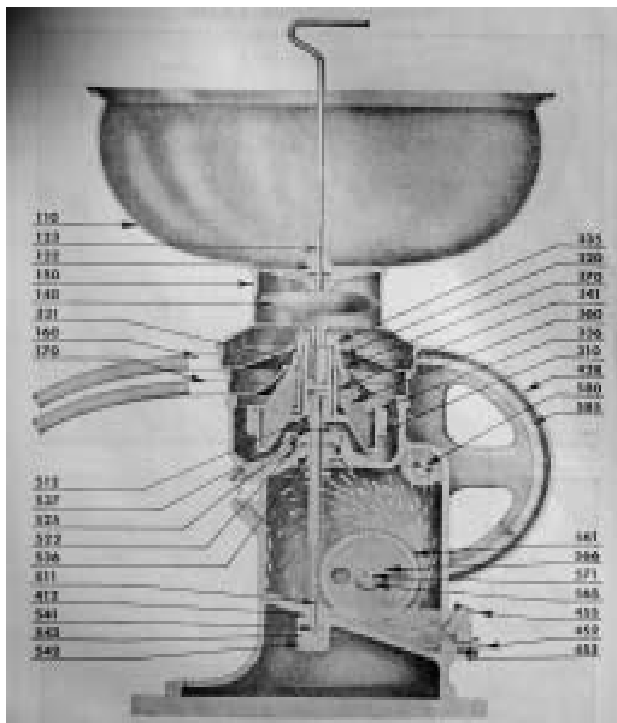
Milka-separaattorin läpileikkaus.
