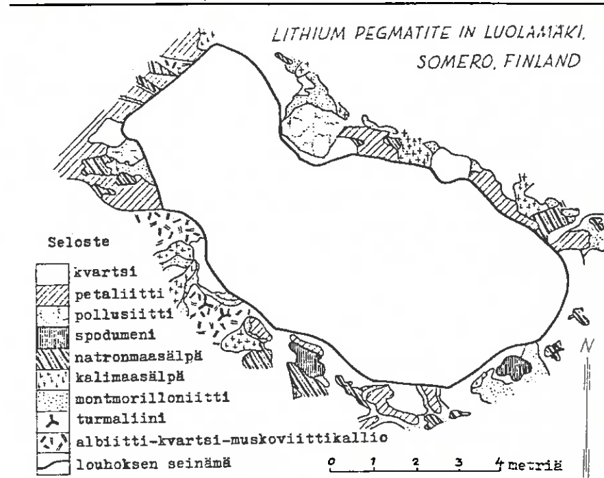
Piirros Luolamäen louhoksesta vaakatasossa Neuvosen ja Vesalon mukaan.
