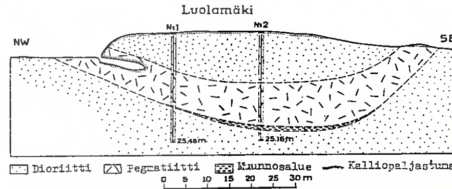
Pystyleikkaus Luolamäen pegmatiittikalliosta Aurolan mukaan. Vasemmalla on vanha louhosluola ja keskellä timanttikairausten reijät.
