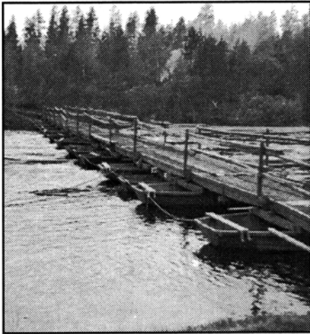
Korpijoen ylityksen yhteydessä oli kuormastoa varten rakennettava silta.
