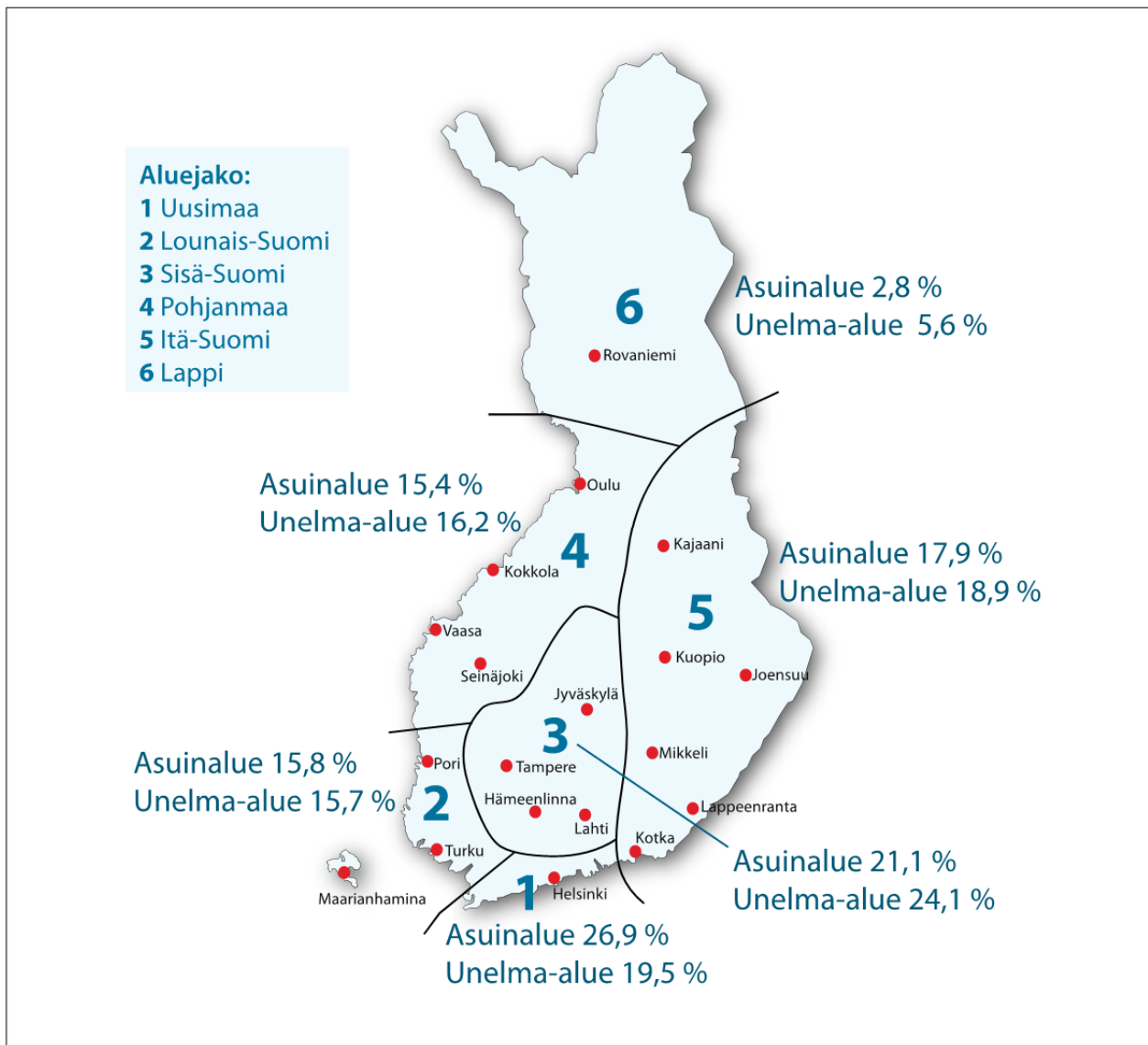
Kuva 39. Alueiden osuudet unelmatulevaisuuksista (n=718) ja vastaajista (n=748).
