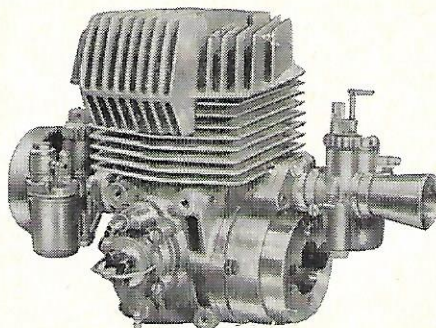
KOMET K 96 Grand Prix
