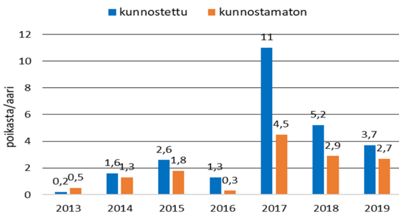
Kuva 23. Vuoksen pääuoman keskimääräinen taimentiheys kunnostetuilla ja kunnostamattomilla koealoilla (Tapaninen M. 2019 Vuoksen kirjanpitokalastus ja sähkökalastustulokset).
