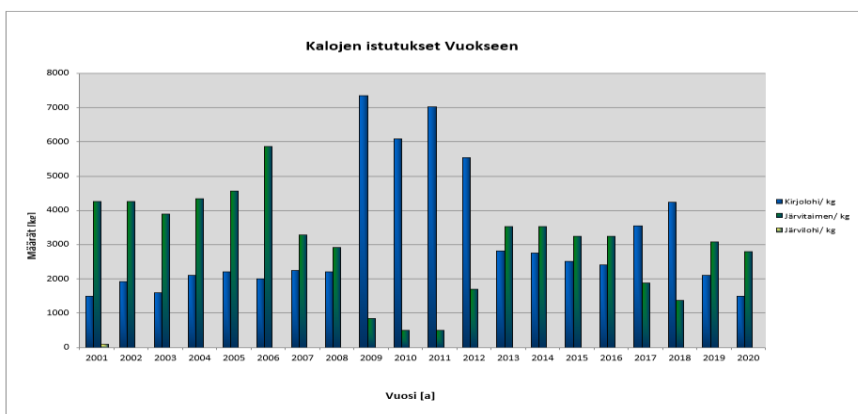
Kuva 22. Kalojen istutukset Vuokseen 2001-2020 (Luonnonvarakeskus. 2021)
