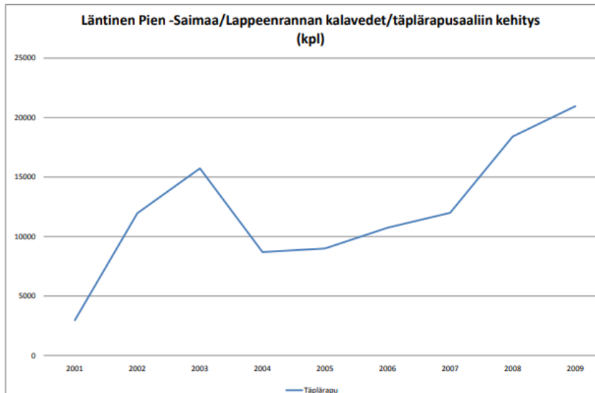
Kuva 16. Täplärapusaaliin kehitys (kpl) Lappeenranta kalavesillä vuosina 2001-2009. (Tiitinen V. 2010)
