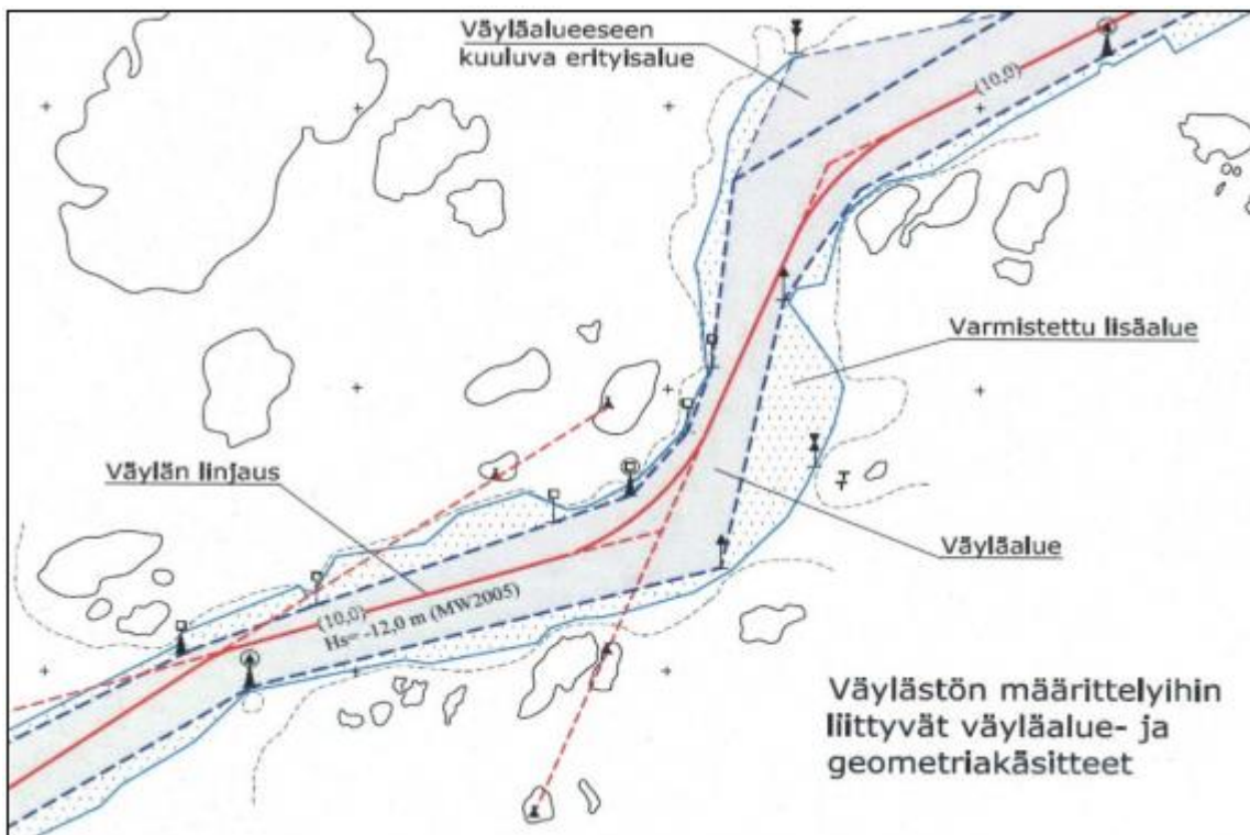
kuva 31. Vesiväylän väyläalue- ja geometriakäsitteet (Liikennevirasto: Vesiväyliin liittyviä käsitteitä, Dnro 1342/610/2005, 31.10.2011)
