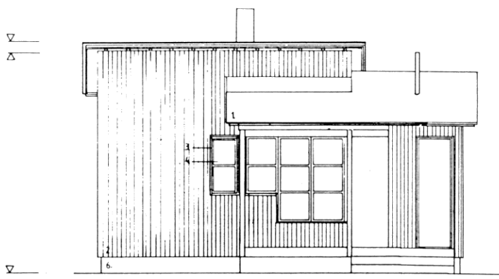
JULKISIVU PUUTARHAAN
