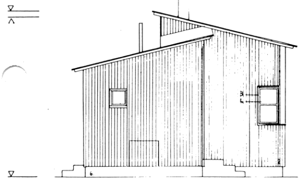
PÄÄTYJULKISIVU
