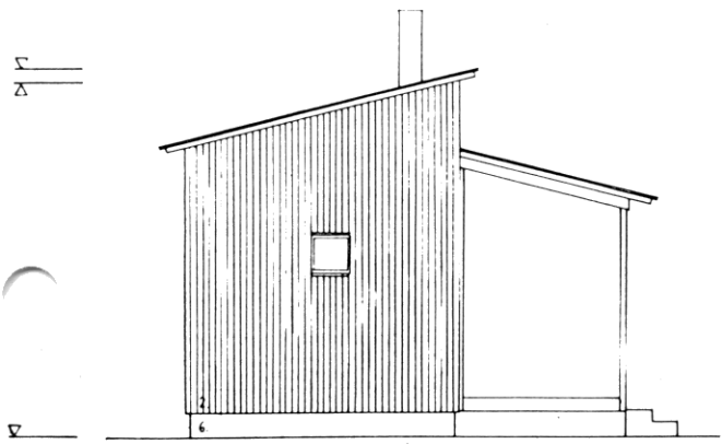
PÄÄTYJULKISIVU
