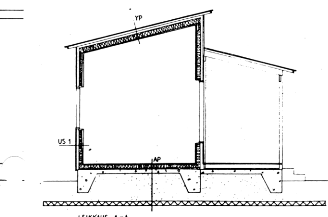
LEIKKAUS A-A
