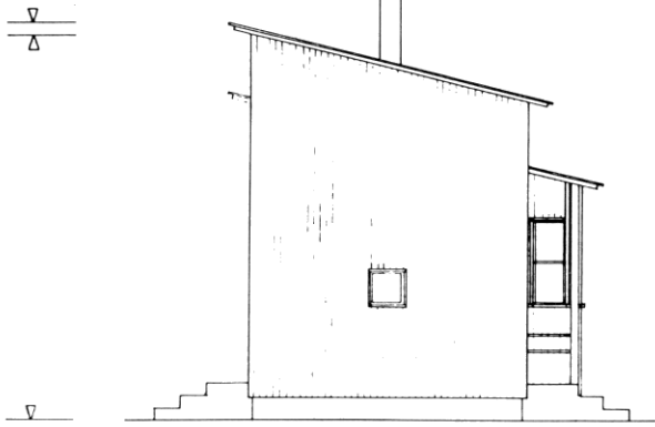
PÄÄTYJULKISIVU
