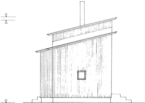
PÄÄTYJULKISIVU
