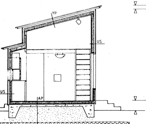
LEIKKAUS A-A
