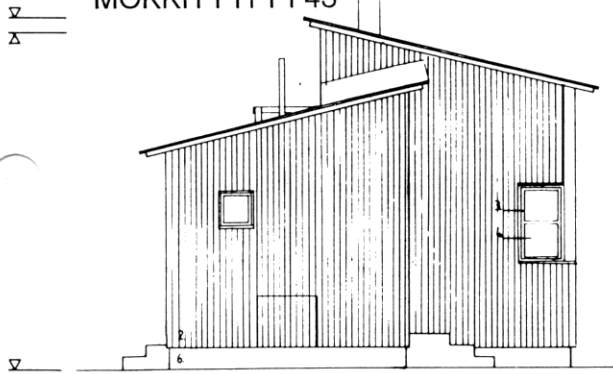
PAÄTYJULKISIVU
