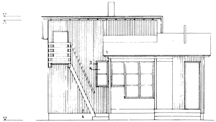
JULKISIVU PUUTARHAAN
