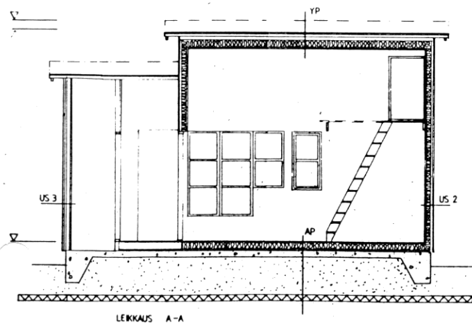
LEKKAUS A-A
