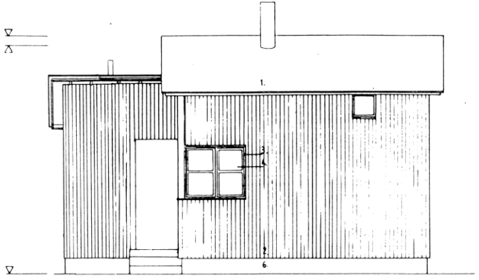
JULKISIVU TIELLE
