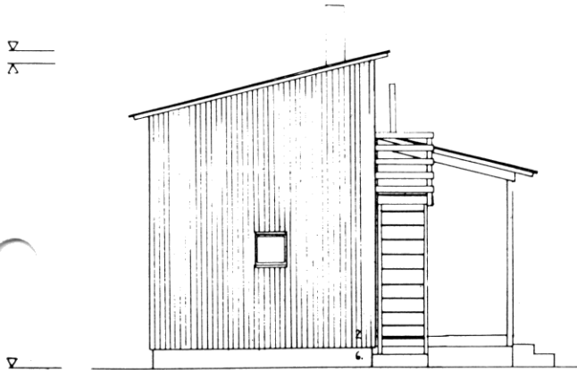
PAÄTYJULKISIVU
