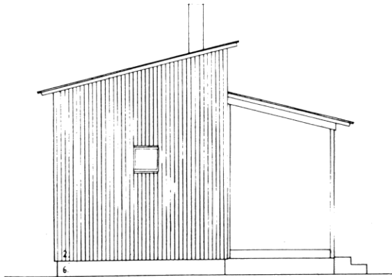
PÄÄTYJULKISIVU
