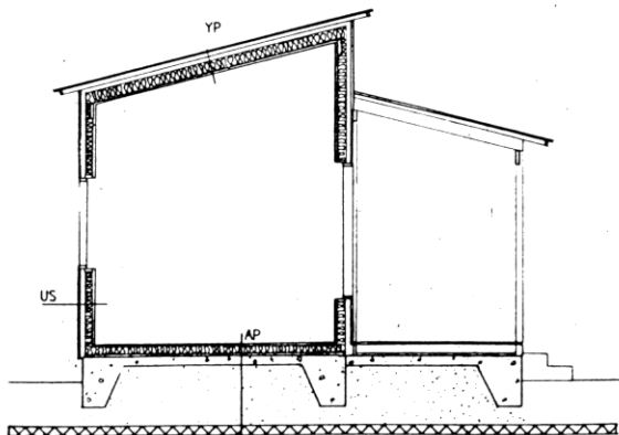
LEIKKAUS A-A
