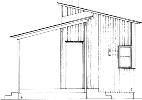
PÄÄTYJULKISIVU
