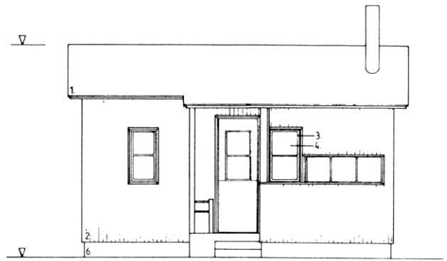
JULKISIVU TIELLE
