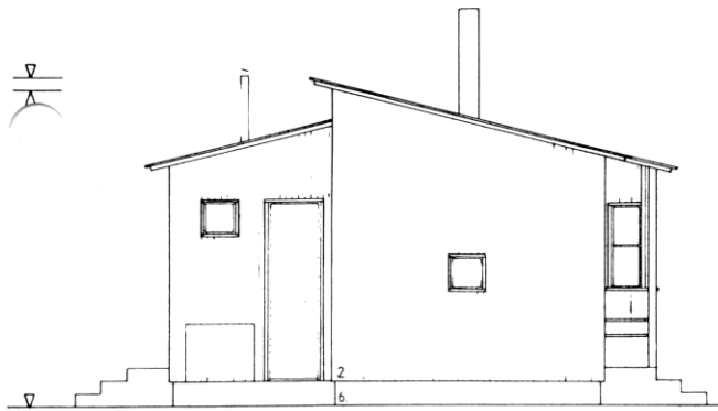
PÄÄTYJULKISIVU
