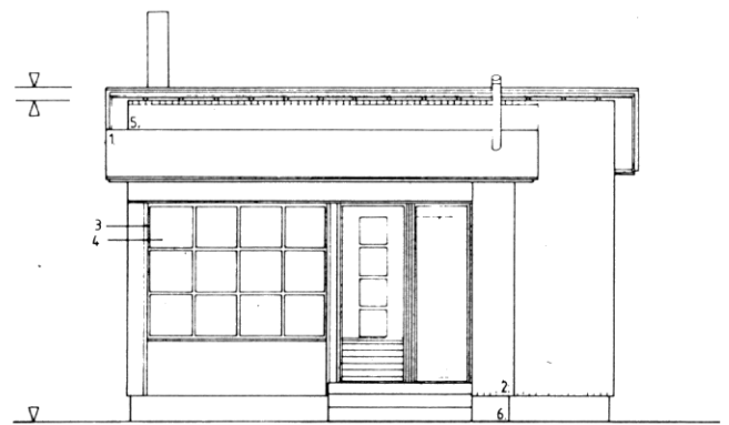
JULKISIVU PUUTARHAAN
