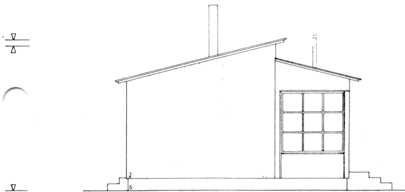
PÄÄTYJULKISIVU
