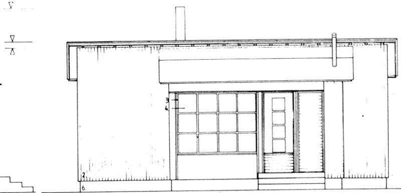
JULKISIVU PUUTARHAAN
