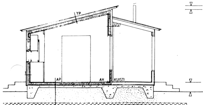
LEIKKAUS A-A
