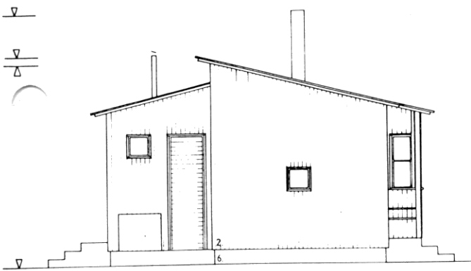
PAATYJULKISIVU
