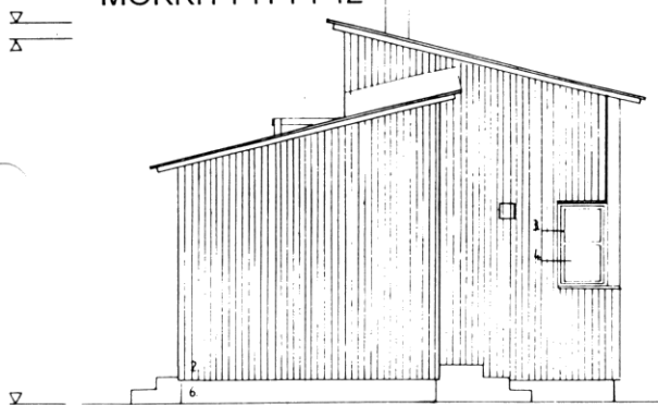
PAÄTYJULKISIVU
