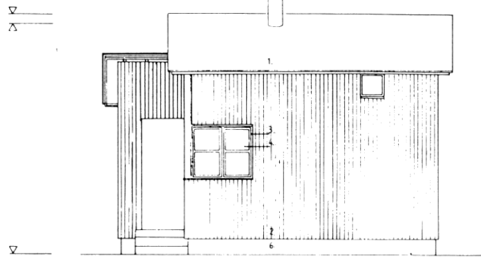
JULKISIVU TIELLE
