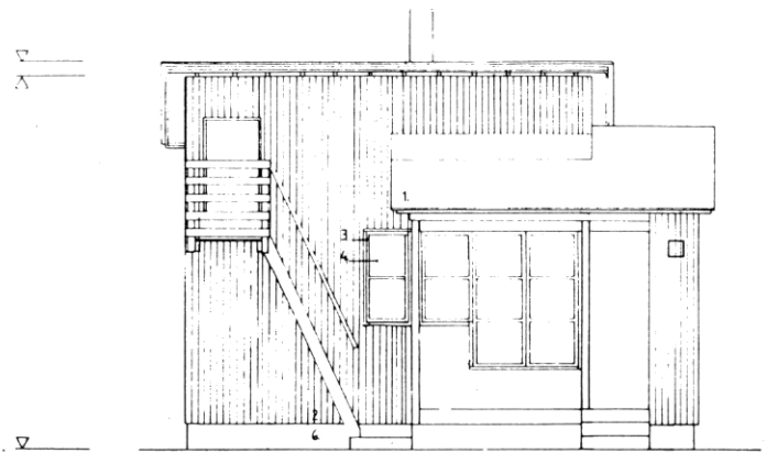
JULKISIVU PUUTARHAAN
