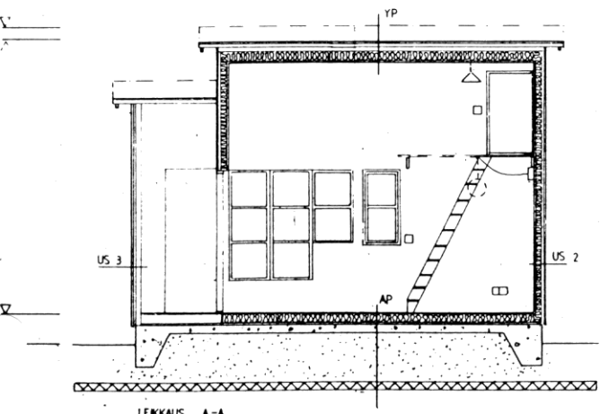
LEIKKAUS A-A
