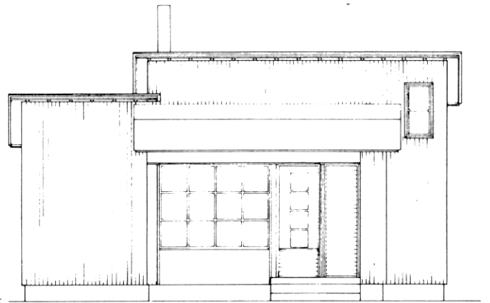
JULKISIVU PUUTARHAAN
