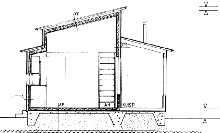
LEIKKAUS A-A
