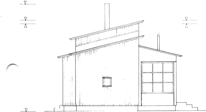
PAATY JULKISIVU
