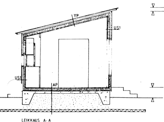
LEIKKAUS A-A
