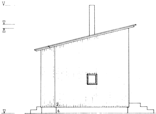
PAATYJULKISIVU
