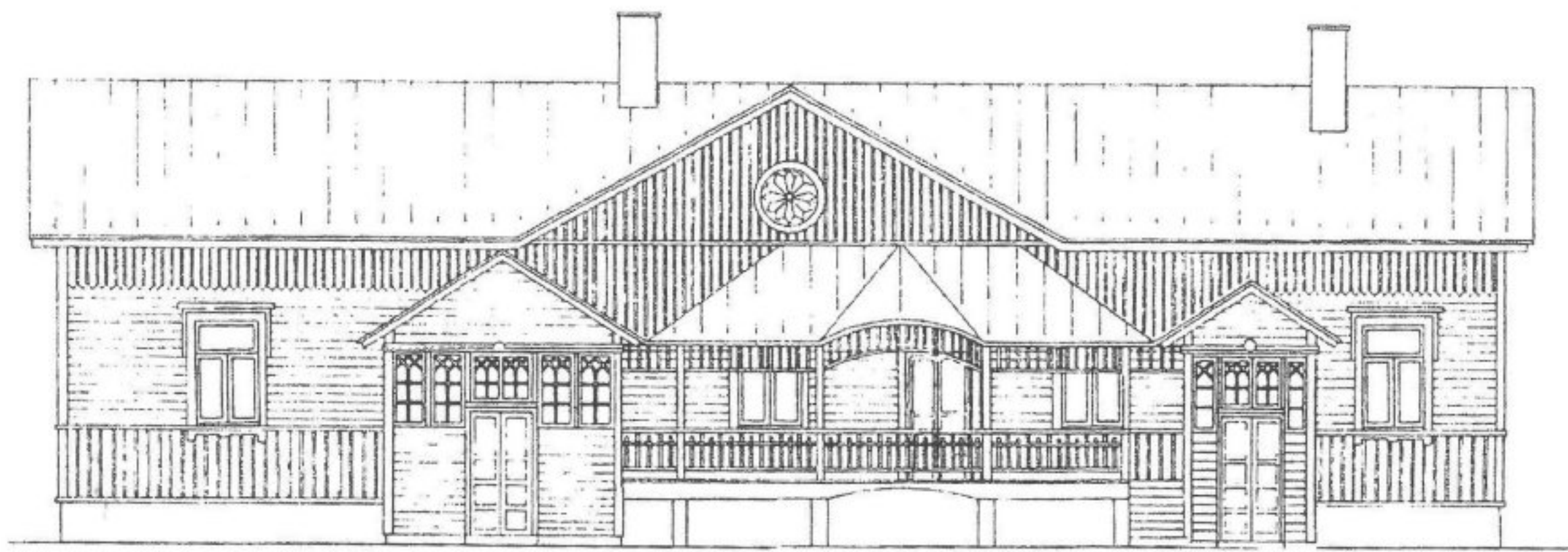
Mikkolan pääjulkisivu terassin valmistuttua ~1918-1922 -uusi avoterassi kuistien väliin -ovi terassille
