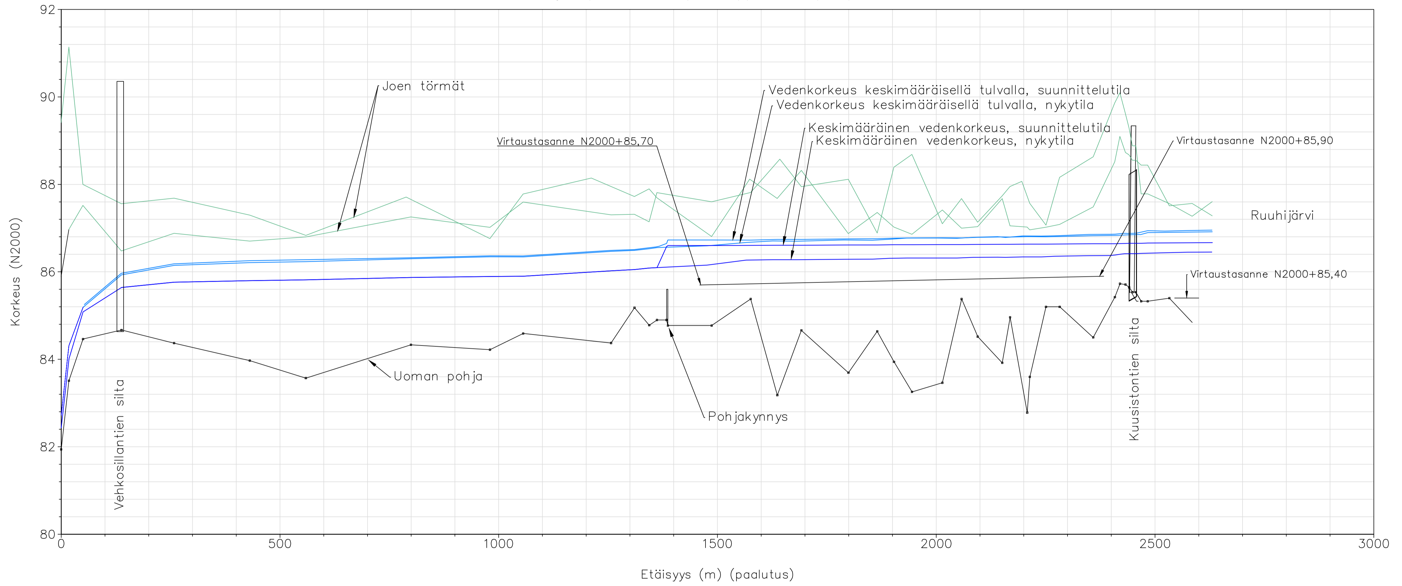
Immilänjoki, pituusleikkaus (korkeus/pituus = 1/100)
