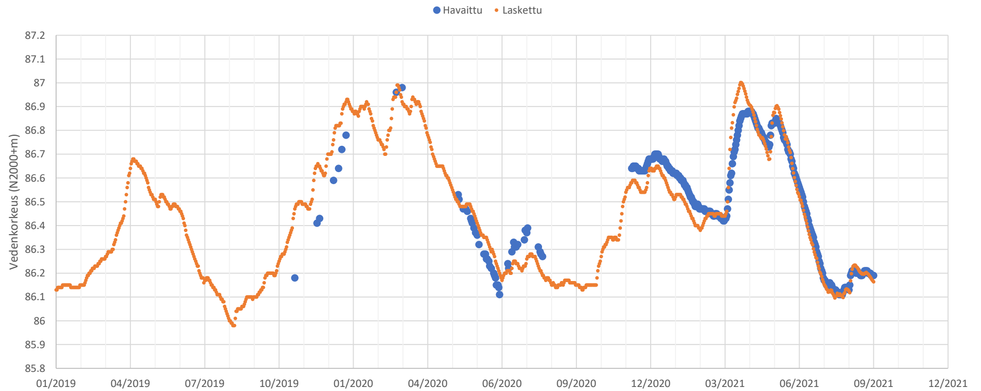
Salajärven ja Ruuhijärven vedenpinnan nosto, havaitut ja lasketut vedenkorkeudet nykytilassa
