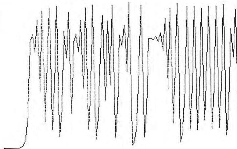
Kuva 5: Populaation koon vaihtelu muuttuu hyvin voimakkaaksi, kun kasvunopeus lähestyy arvoa 4. Vaihtelu näyttää jo täysin säännöttömältä, kaoottiselta.
