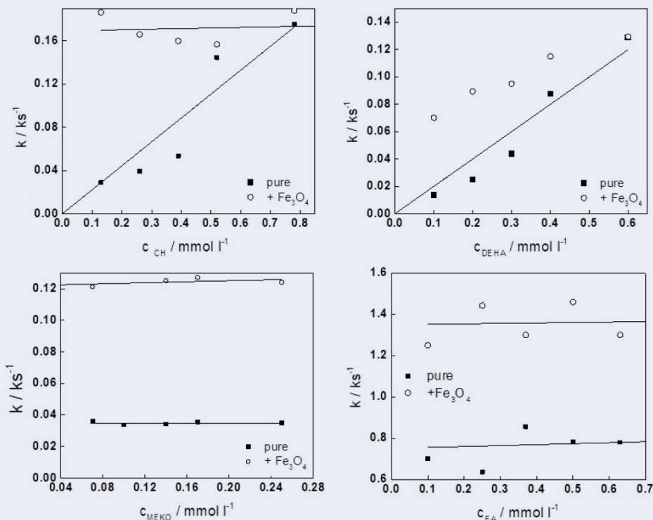
Kuva 3. Huoneenlämpötilassa määritetyt reaktiovakio k :n arvot eri hapensyöjäkemikaaleille (CH = karbohydraatti, DEHA = dietyylihydroksyliamiini, MEKO = metyylietyyliketoni ja EA = erytorbiinihappo) magnetiittisäyksellä ja ilman. [5]
