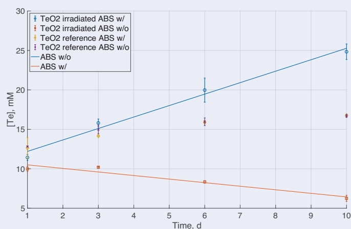
Kuva 2. Telluurin liukoisuus säteilytysajan funktiona sumpppiin lisätyllä tiosulfaattilla (sininen, o) ja tiosulfaatin kanssa (oranssi, +). Keskimäiset datapisteet (keltainen, violetti) esittävät referenssitapauksia säteilyttämättömissä liuoksissa.
