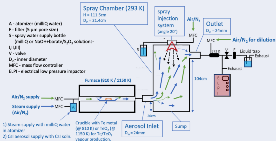
Kuva 6. Koelaitteisto, jota käytettiin ruiskutusjärjestelmän tehokkuuden testaamiseen.
